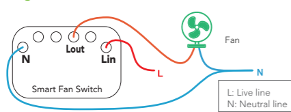
Diagram 2: For fan control
